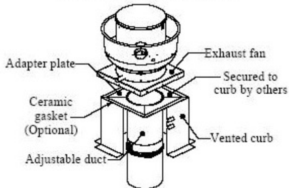
Fig. 7 – Fan Adapter Plate
